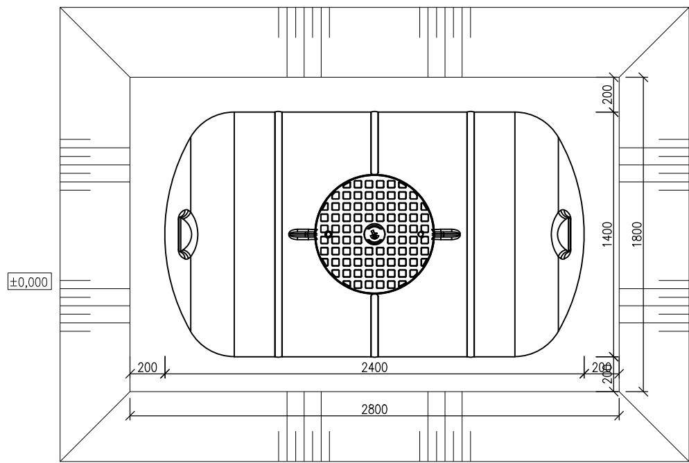
PŮDORYS
